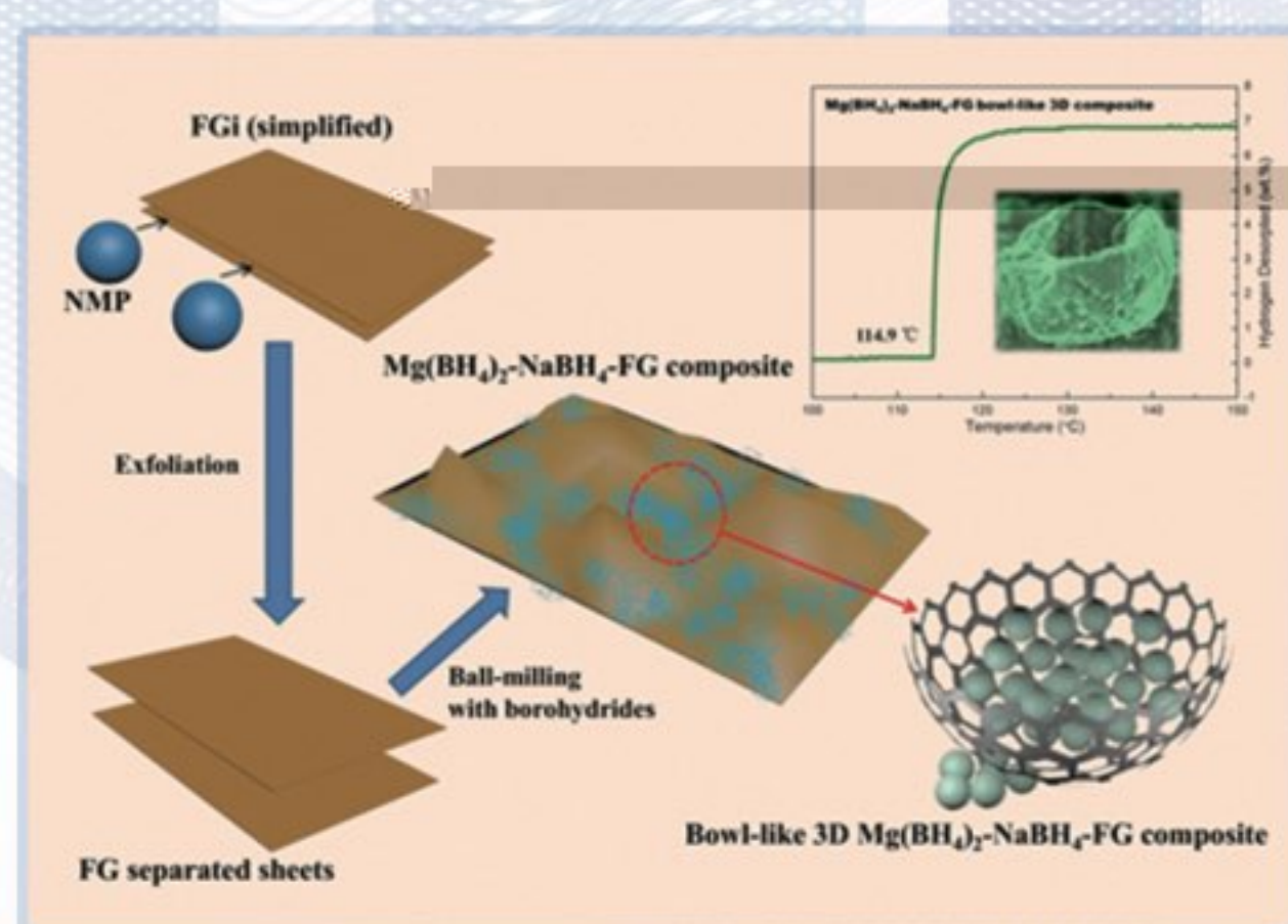
近室温放氢的Mg(BH 4 ) 2 -NaBH 4 -FG储氢材料
